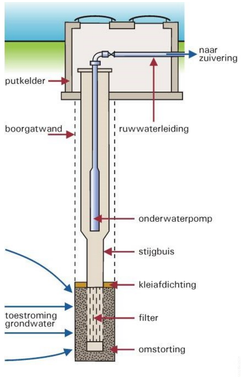
Doorsnede pompput
